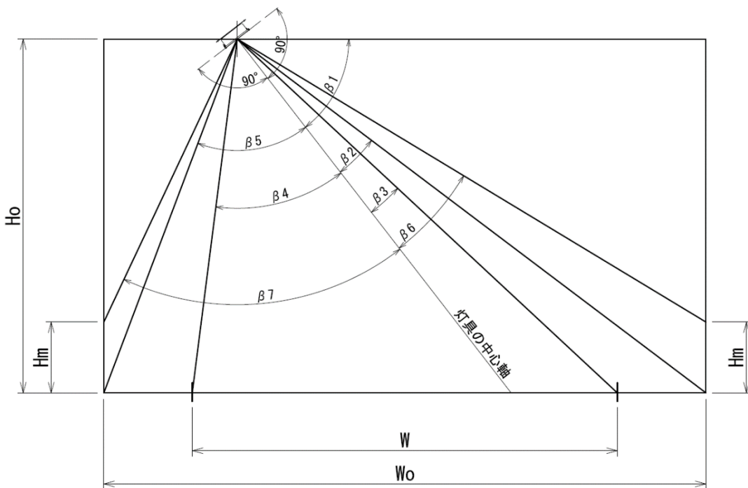
(a) トンネル断面と角度の取り方
